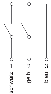
Elektrisches Schema
